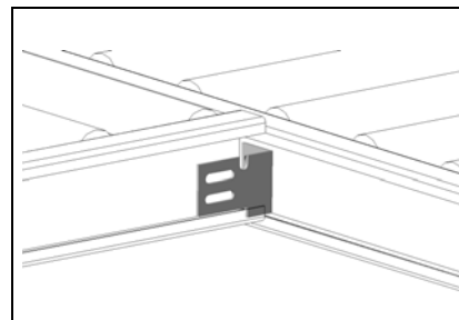
AX100 – Fästvinkel, tvärställd bana *
