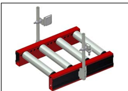
AX100 – Givarfäste utsida spant Typ GFU *
