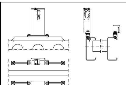
PA1500 – Fotocell och reflex med fästen
