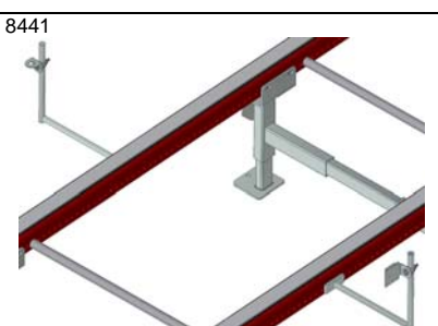
KRT100 – Givarfästen utsida spant
