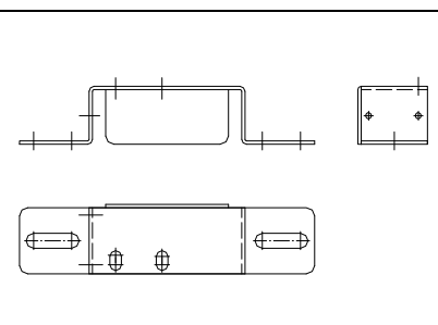
AX100 – Fotocellfäste
