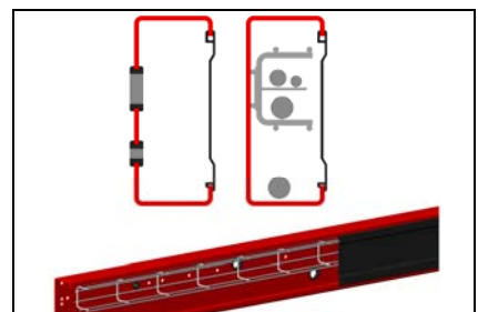
PA1500 – Kabelkanal i spant
