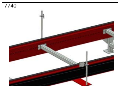
PA1500 – Fästen för fotocell och reflex. Till kedjetransportör
