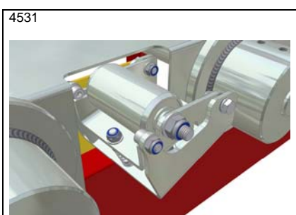
Flänshjulbana - Indikeringsrulle
