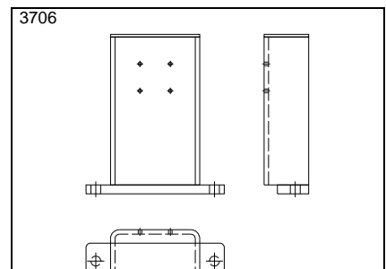
PA1500 – Fotocellfäste
