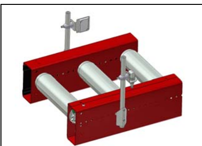
PA1500 – Givarfäste utsida spant Typ GFU *
