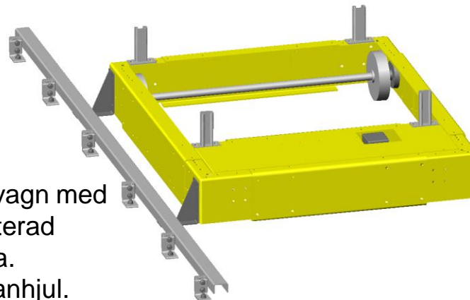
Transfervagn med flänshjul. Rälsgående.
