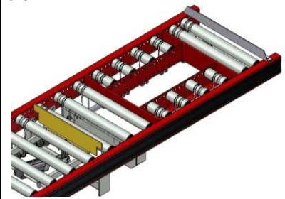
AX100 – Rullbana med urtag för lyftanordning
