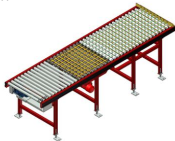
FR100 – Rullbana. Remmar mellan rullsegment hindrar att kartongflikar går ner mellan rullar
