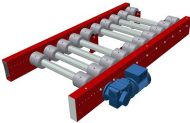
KE500 – Rullbana, fast driven. Förstärkt med stålhylsor för transport av stålgoods
