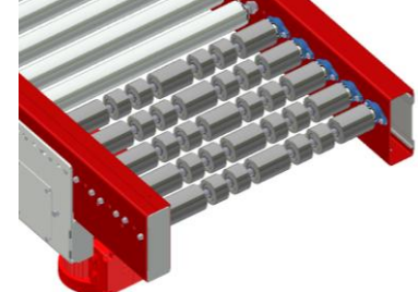
KE500 – Rullbana med urtag i rullar för robotens gripdon
