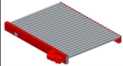
KE500 – Rullbana, fast driven. Med kraftigare spant för tungt gods
