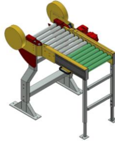
KE500 – Grind, driven, med motvikt. Fristående, med en kort fast rullbana
