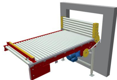
KE100 – Uppfällbar rullbana. Motordriven uppfällning
