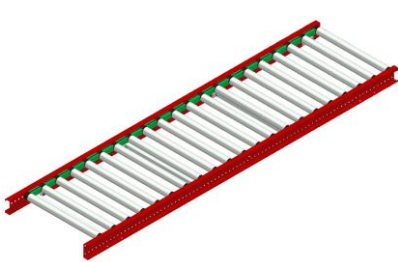
ZP100 – Driven rullbana med 24 V drivna rullar för trycklös ackumulering. Poly-V remmar
