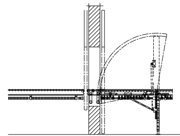
AX100 – Grind vid brandvägg
