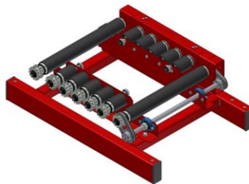
KE500 – Urtag i rullbana vid arbetsstation
