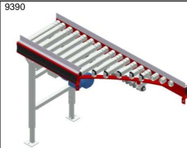
AX100 – Vinkelanslutning mot kurva
