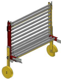
AX100 – Grind, driven, med motvikt
