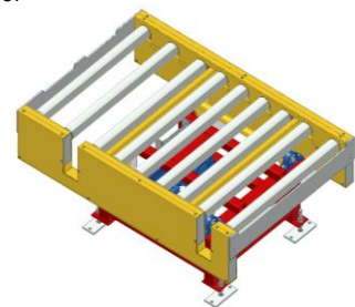
PA1500 – Høj- och sänkbar rullbana med elektrisk lyftrörelse
