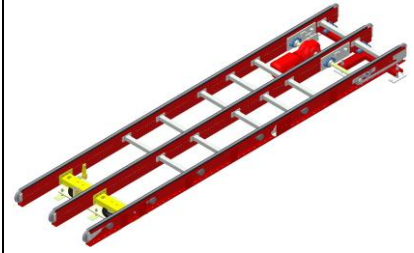
PA1500 – Tiltbar kedjetransp., lågbyggd. TH 300 mm. Förstärkt för lång längd och last 1500 kg
