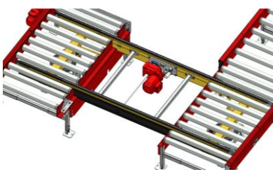
PA1500 – Kedjetransportör, separat tiltbar i vardera änden
