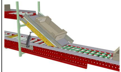
FR100 – Tiltbar slisk för att sammanföra flödet av tomlådor från 2 nivåer
