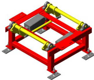
PA1500 – Lyftenhet, pneumatisk Typ LP *
