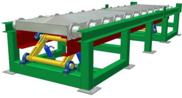
Flänshjulbana – Høj- och sänkbar transportör, hydraulisk. 3000 kg
