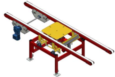
KRT100 – Høj- och sänkbar kuggremstransportör med høj- och sänkbar vändplatta
