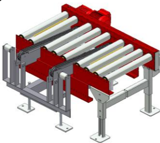
KE500 – Tiltbar kedjetransportör
