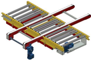
FR100 – Høj- och sänkbar rullbana med kuggremstransportör som växel
