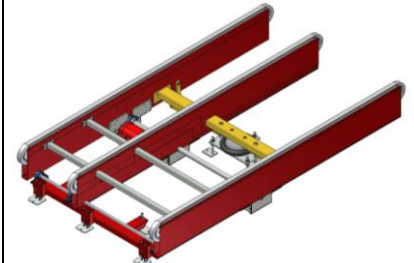
PA1500 – Tiltbar kedjetransportör, 3 kedjor, 2½" plastkedja
