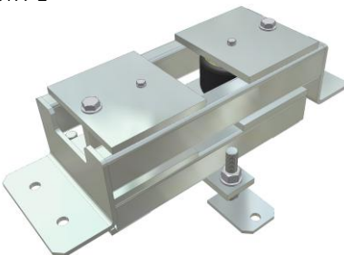
PA1500 – Tilt- och lyftenhet med bälg för låga transporthöjder
