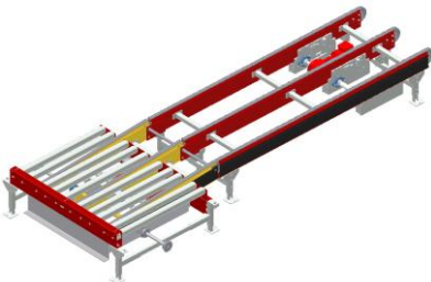
PA1500 – Kedjetransportör med tiltbar ände. Motordriven lyftrörelse
