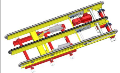
PA1500 – Tiltbar kedjetransportör. Lyftrörelse med cylindrar
