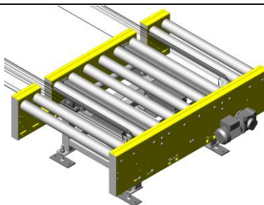
PA1500 – Høj- och sänkbar rullbana, pneumatisk, Typ HSR *
