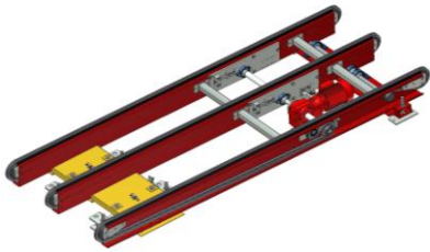
PA1500 – Tiltbar kedjetransportör, 3-strängad, lågbyggd. TH 240 mm
