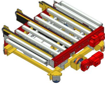
PA1500 – Vridbar rullbana med hjul, med vinkelväxel
