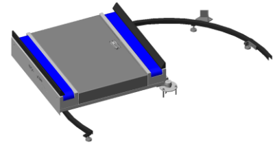
PA1500 Rostfritt – Svängmodul, driven, med 2-strängad plastlamelltransportör
