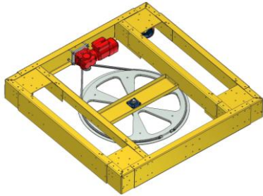
PA1500 – Vridmodul för stor, tung last, 2600 kg
