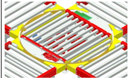
PA1500 – Vridbar rullbana. Stödrullar för godset, med skydd för minskad klämrisik
