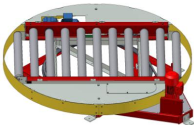
PA1500 – Vridbar rullbana, lågbyggd. TH 250 mm
