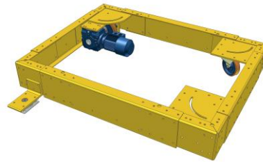
PA1500 – Svängmodul Typ SM *. Driven
