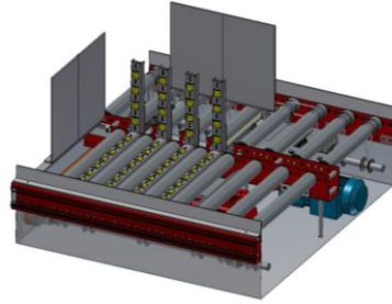
AX100 – Vertikalvändare för att vända godset 90° åt sidan
