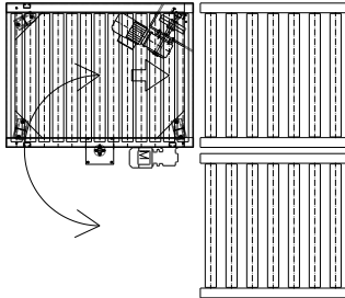
PA1500 – Svängmodul med rullbana använd för att växla över godset från en bana till en annan
