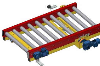
PA1500 – Svängbar rullbana. Lågbyggd, TH 250 mm
