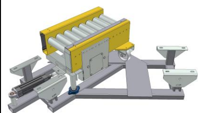
KE500 – Svängmodul, pneumatisk
