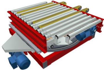
AX100 – Vridmodul med rullbana och vinkelväxel
