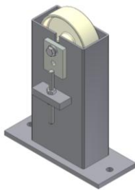
PA1500 – Stödhjul till vridbar rullbana. Minsta TH 400 mm
