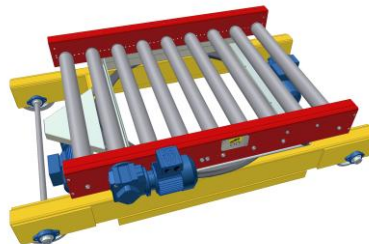
PA1500 – Transfervagn på räl med vridbar rullbana, lågbyggd. TH 430 mm
