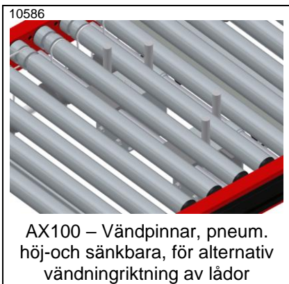
AX100 – Vändpinne, pneumatiskt höj- och sänkbar
