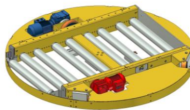
PA1500 – Vridbar rullbana, lågbyggd med hjul. TH 115 mm
