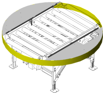
PA1500 – Klämskyddsring till vridbar rullbana *
