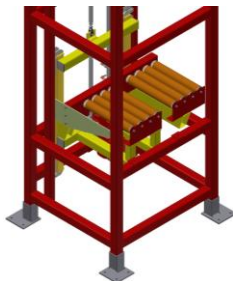
KE500 – Godsliftare med rullbana med urtag för kedjetransportörs kedjesträng
