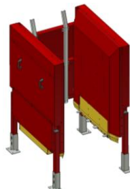
PA1500 – Pallmagasin som hanterar helpall eller 2 halvpall som står efter varandra
