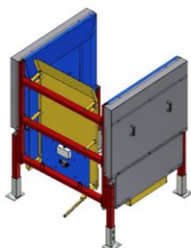
PA1500 – Pallmagasin med manuellt ställbar rygg för 3 olika pallstorlekar
