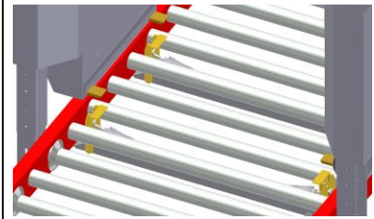
PA1500 – Pneumatisk hållare för delning av pallar som fryst ihop
