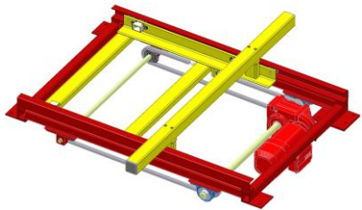
PA1500 – Pusher för uppriktning av pall. Motordriven
