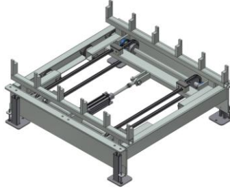
PA1500 – Pallcentrering med fingrar
