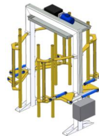
PA1500 – Pallriktare, hydraulisk. Slutet läge
