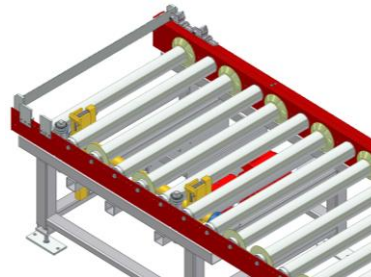
PA1500 – Uppriktning och fixering av stålrack vid robot. Motordriven
