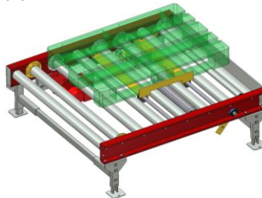
PA1500 – Pneumatisk orientering och låsning av pall i sidled
