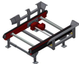
PA1500 – Pallinstyrning, kedjetransportör. Hämtning och lämning från kort- och långsidan
