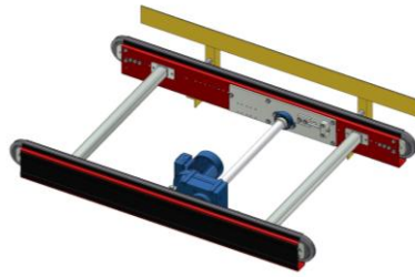
PA1500 – Sidstyrning, kedjetransportör
