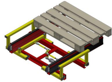
PA1500 – Pallcentrering i kedjetransportör
