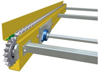
PA1500 – Sidstyrning, kedjetransportör
