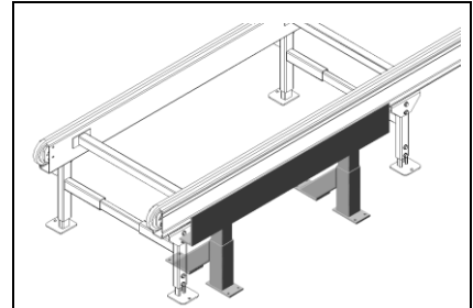
PA1500 – Truckpåkörningsskydd Typ TPK *
